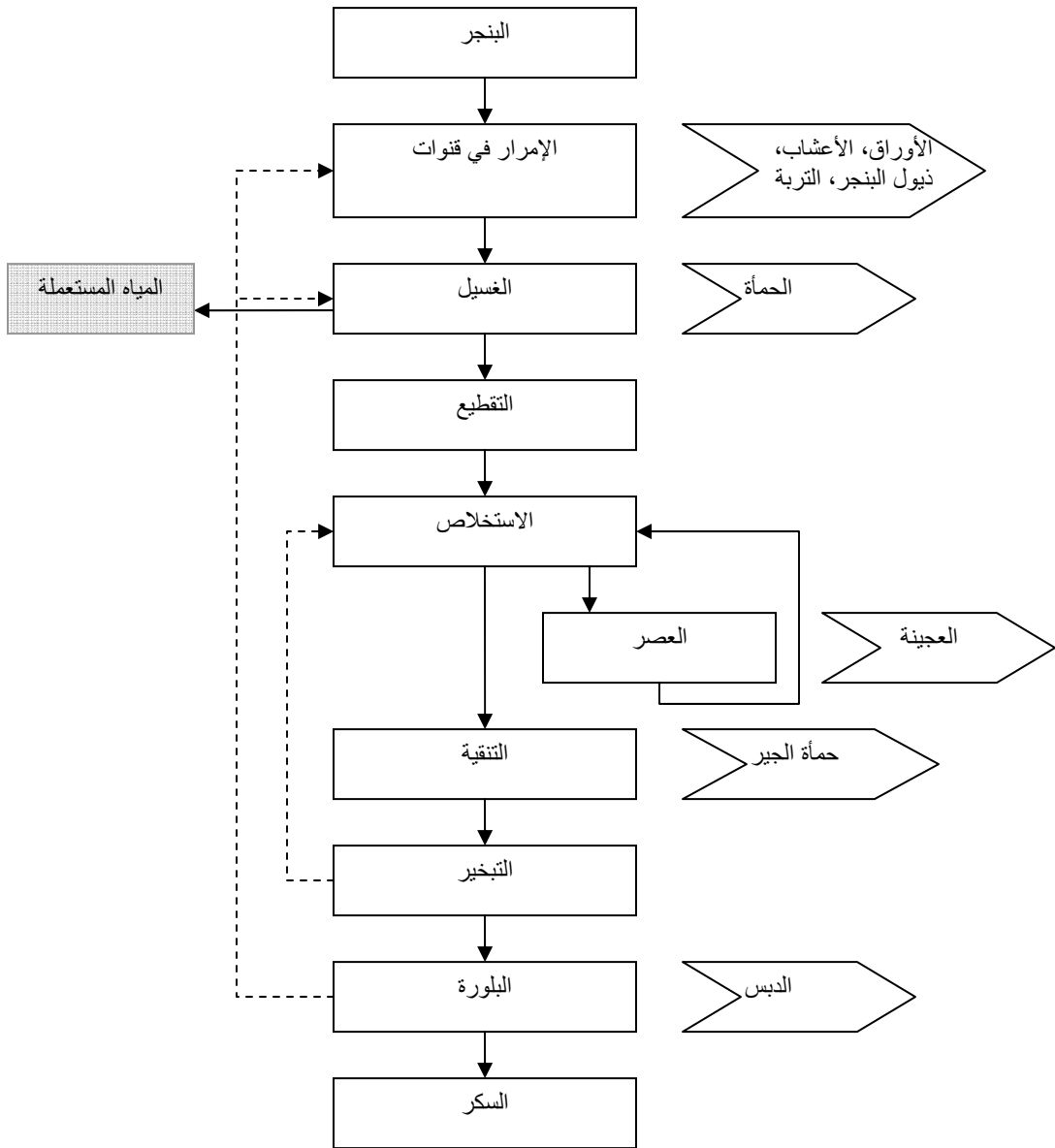
الشكل ألف-1: تصنيع السكر من البنجر
