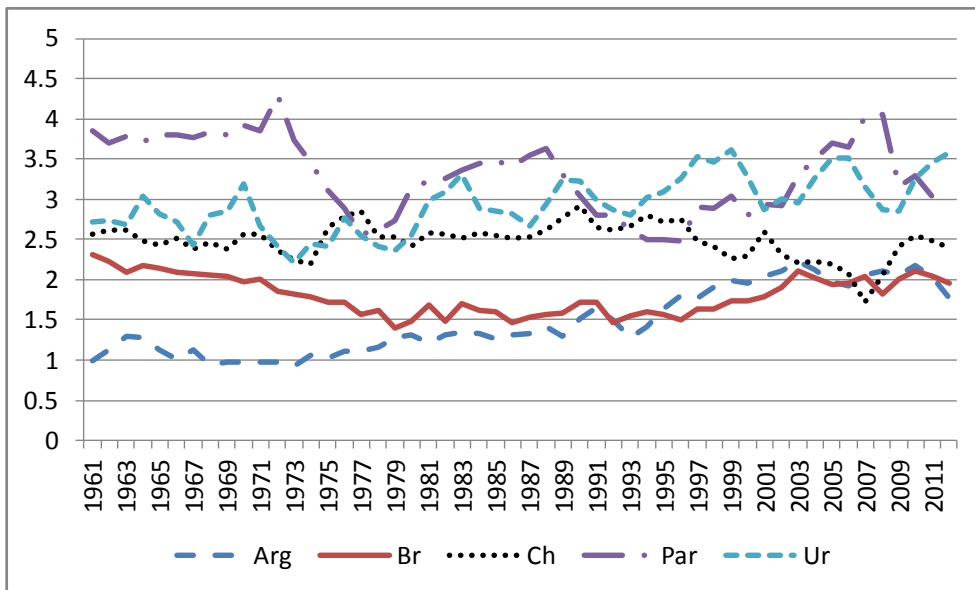
Gráfico 25. Índices de PTF Agropecuaria 1961-2012
