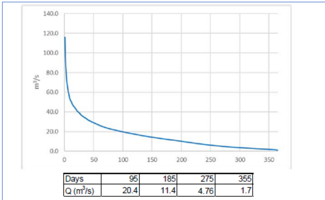
Gambar 6. Kurva Durasi Aliran Sungai Cisokan di Bendungan Bawah (disintesis dari Stasiun Manglid)
