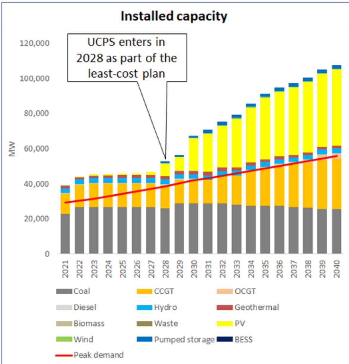
Gambar 9. Rencana Pembangunan Jangka Panjang Sistem Jawa-Bali
