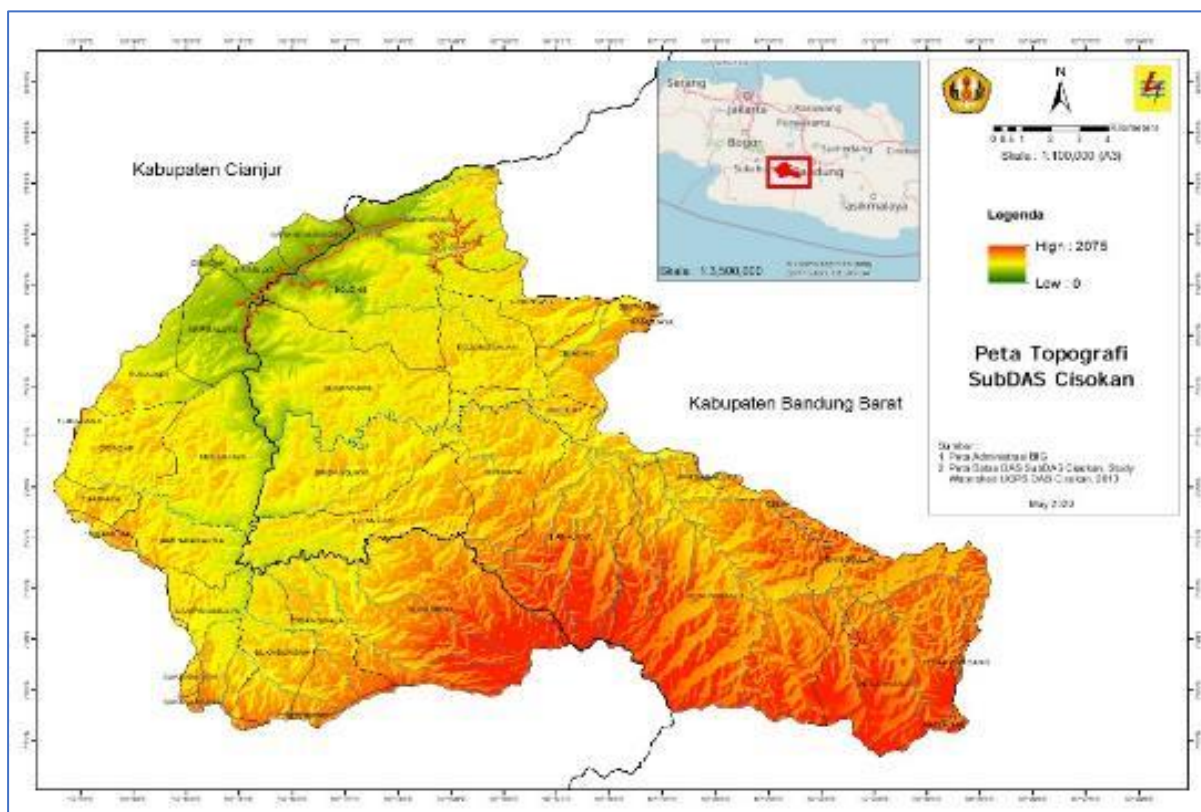
Gambar 3. Topografi DAS Cisokan, bagian dataran rendah ditunjukkan dengan warna hijau merupakan tempat proyek UCPS akan dikembangkan dan warna merah merupakan pegunungan yang lebih tinggi merupakan lokasi Sungai Cisokan berasal.
