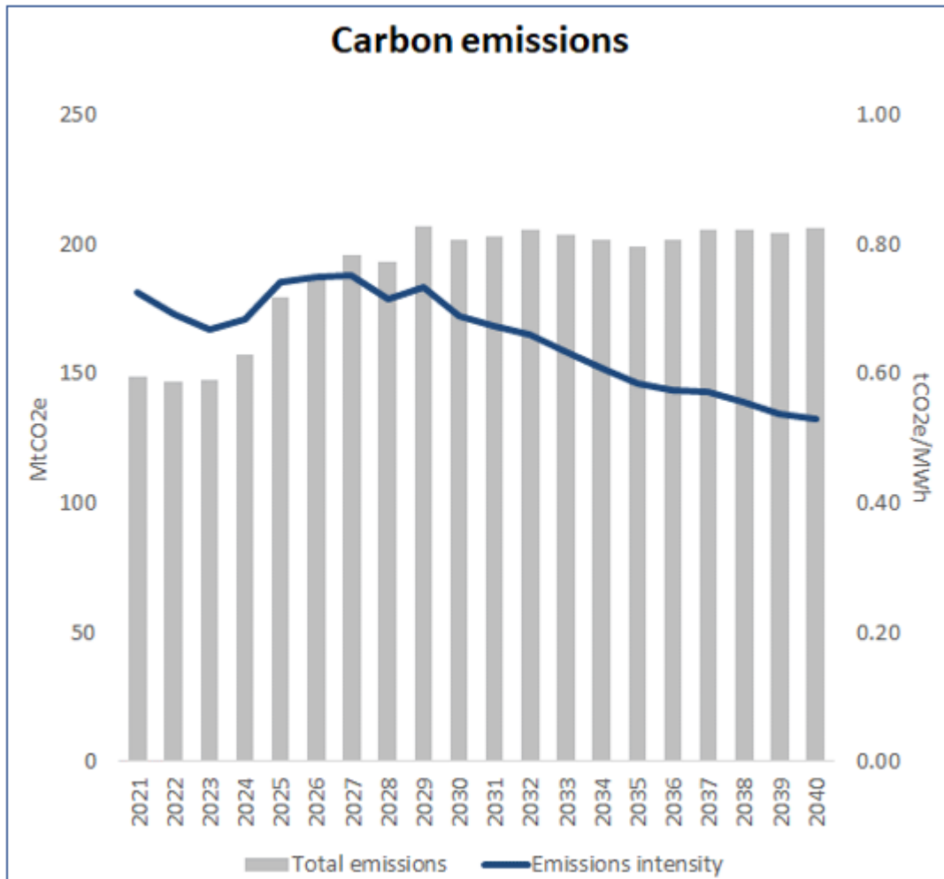
Gambar 10. Intensitas Emisi Sistem Jawa-Bali
