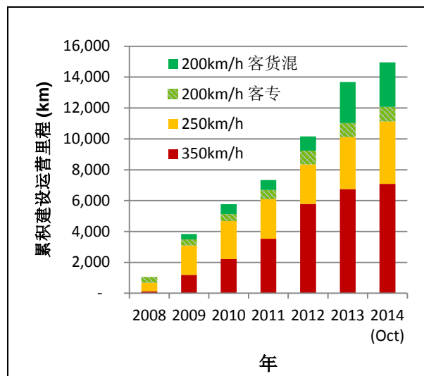
图 1：2008-2014 年 10 月中国高铁及速度为 200 公里/小时线路长度 (来源：中国交通年鉴，中国铁道年鉴和中国铁路总公司计划统计部)
