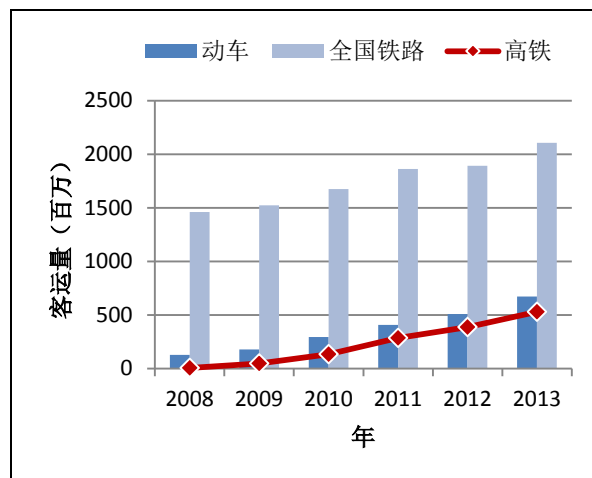
图 3: 全国铁路、动车和高铁线路客运量 (数据来源: 2008-2012 年中国统计年鉴数据; 2013 年中国铁路总公司计划统计部)
