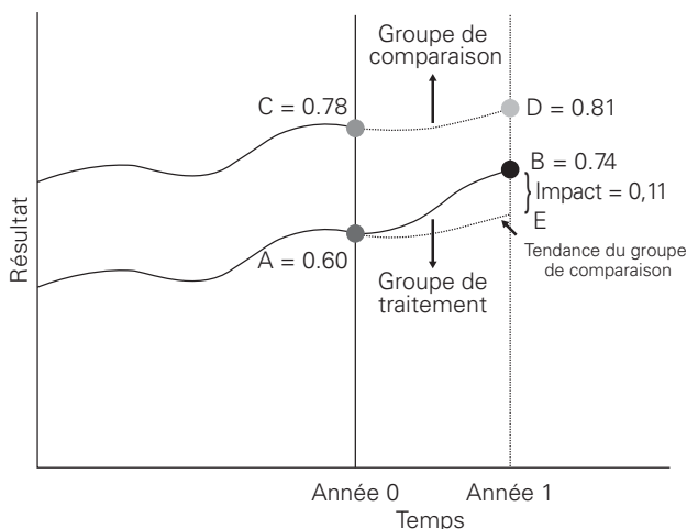
Figure 6.1 Double différence
